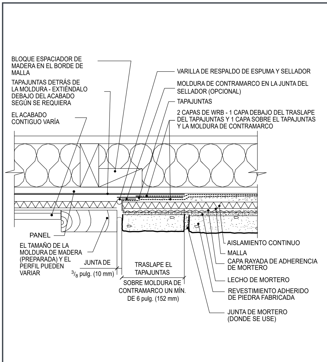
Figura 12b. Transición vertical sobre aislamiento continuo
