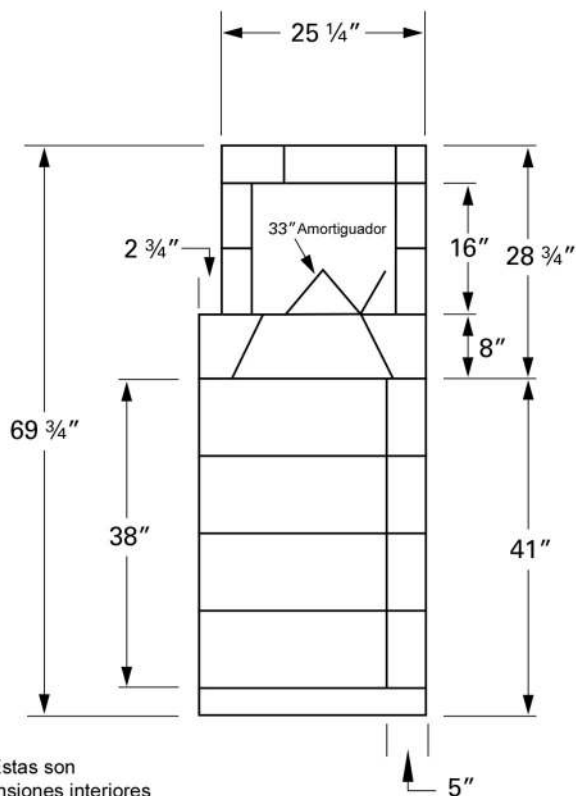
Vista lateral
