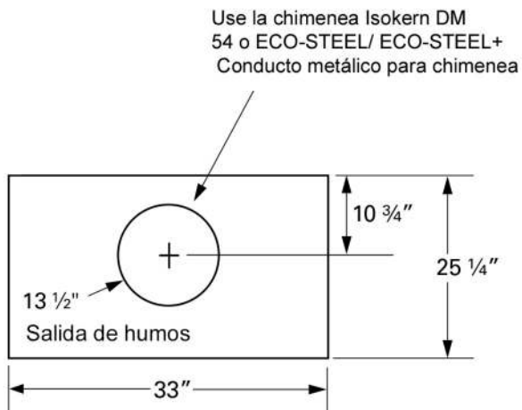
Vista Superior
